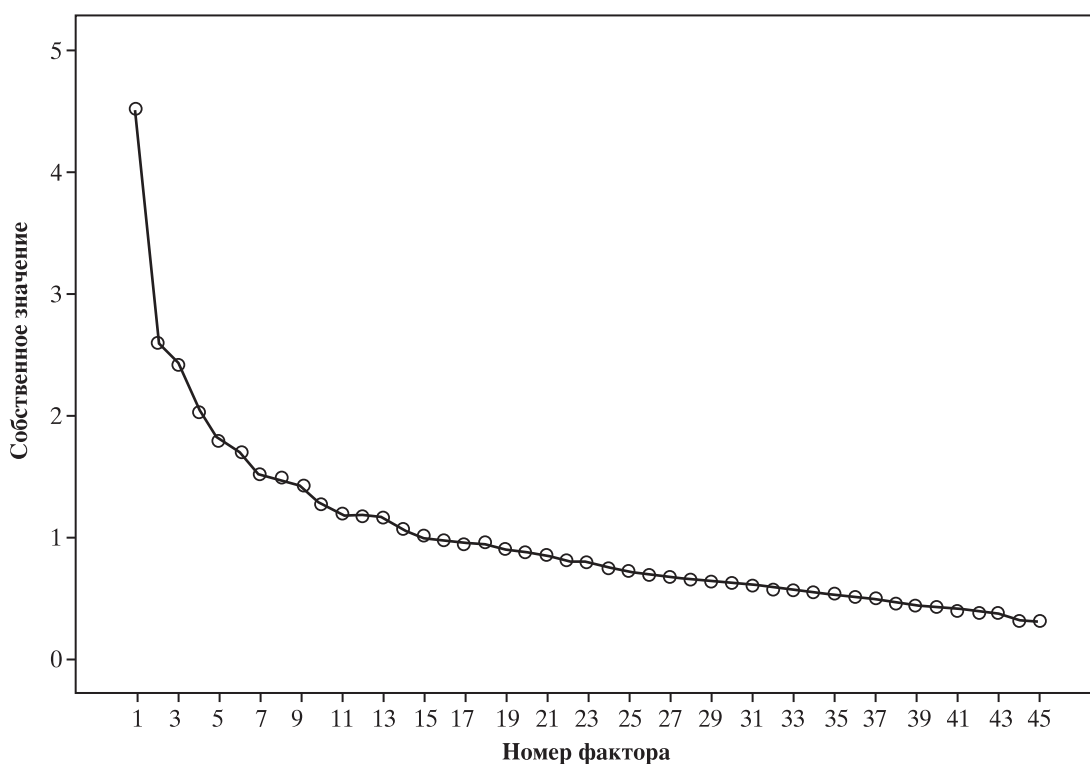
Рис. График-оська для факторизации опросника ШПР (факторизация методом главных осей; вращение Промакс с нормализацией Кайзера).
